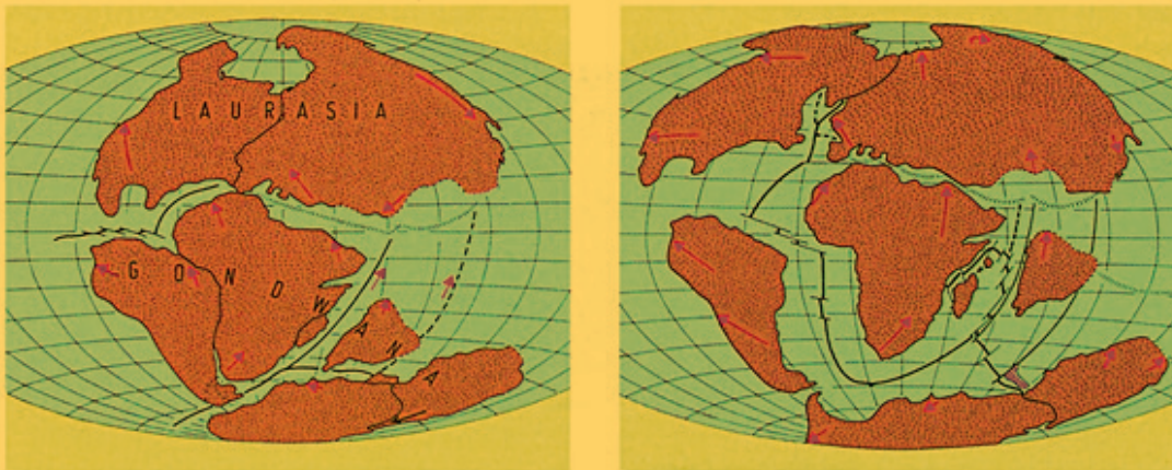
Abb. 1 Lage der Kontinente a) am Ende der Triaszeit vor etwa 180 Millionen Jahren b) am Ende der Kreidezeit vor etwa 70 Millionen Jahren (Pfeile: Bewegungsrichtung der Kontinente)
